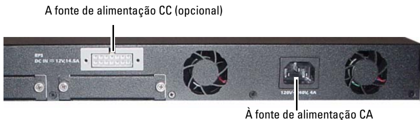
Figura 1-15. Conexão de energia CA e CC ao comutador
