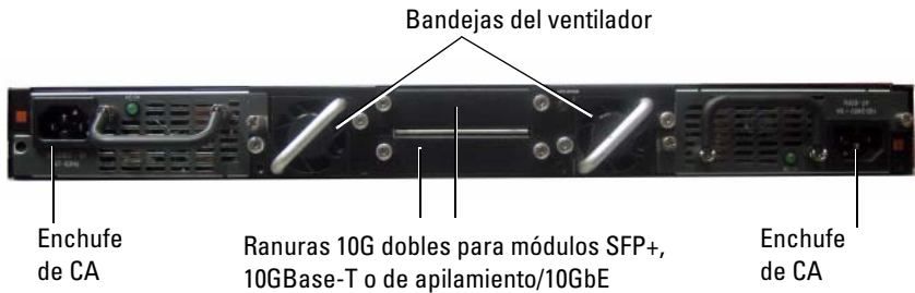
Ilustración 1-10. Panel posterior de PC7048R
